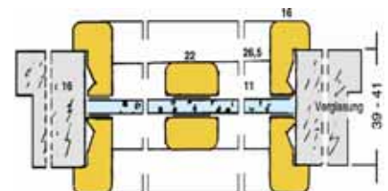
Skizze Flachprofil vom Vorsetz-Sprossenrahmen-Satz flach
