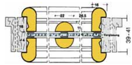
Skizze Rundprofil vom Vorsetz-Sprossenrahmen-Satz rund
